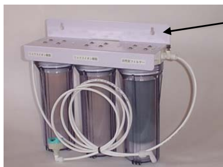
3本吊下げ型 参考写真 (イオン樹脂、活性炭 装入例)
